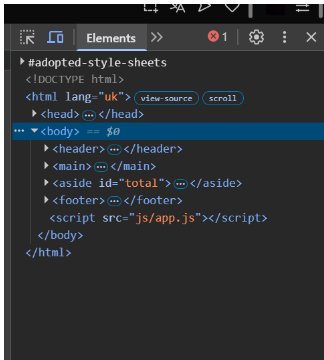
Рис. 3 Вигляд дерева DOM (відповідає задуму)
